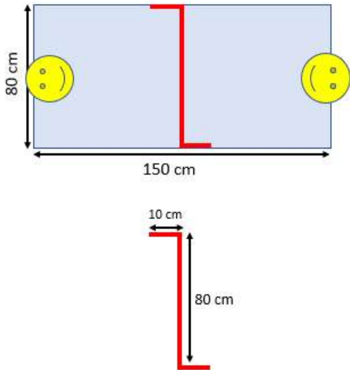
Construcción de barrera, diseño digital
