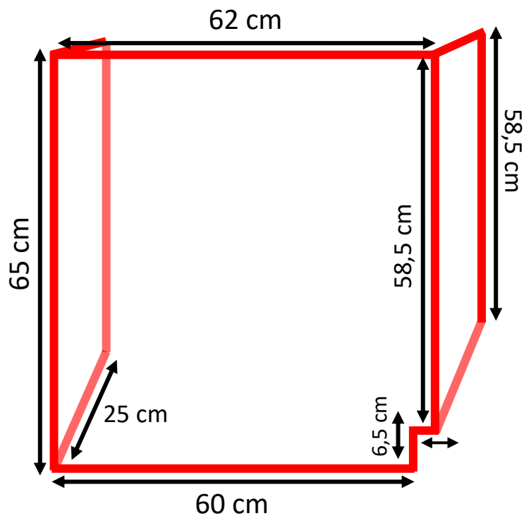
Construcción de barrera, diseño digital
